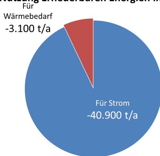
Abbildung 5-3: Einsparung an CO 2 e-Emissionen im Jahr 2022 durch den Einsatz Erneuerbarer Energien
