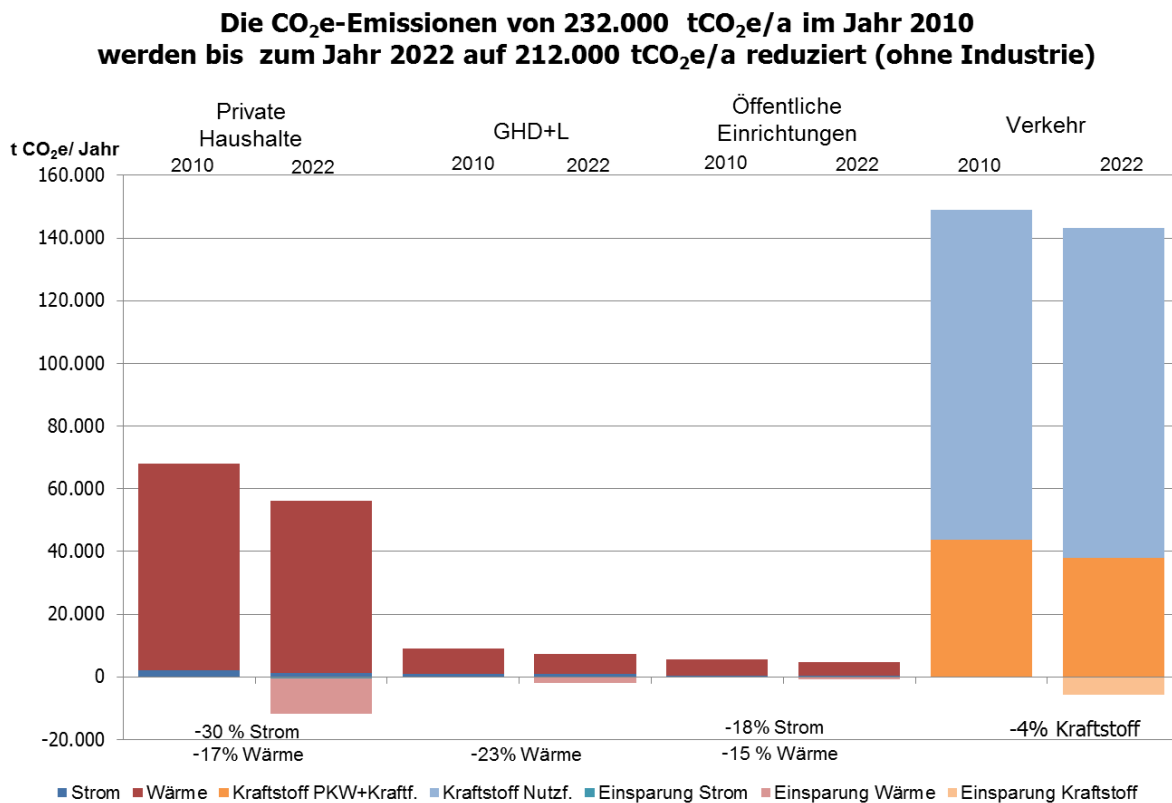
Abbildung 4-22: Entwicklung der CO 2 e-Emissionen in Ingelheim 2010-2022
