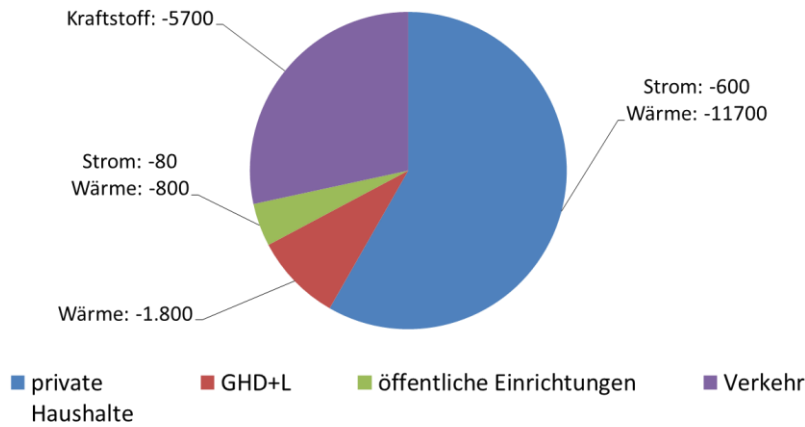
Abbildung 5-4: Aufteilung der Emissionsminderung durch Effizienzmaßnahmen
